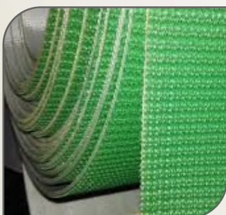
Rough Top Green 5 mm Thick per DIN 22102
